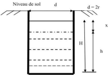
Figure 7 : Mesure de la perméabilité par méthode de Porchet (Houngkpetin, 2003)
