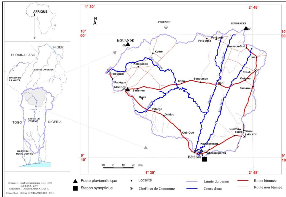
Figure 1: Situation géographique du bassin de l'Ouémé à Bétérrou
