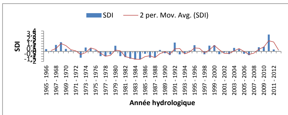
Figure 5: Indices annuels de sécheresse hydrologique sur le bassin de l'Ouémé à Bétérou
