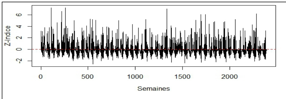
Figure 7: Indices hebdomadaires de sécheresse agricole (Z Indice)
