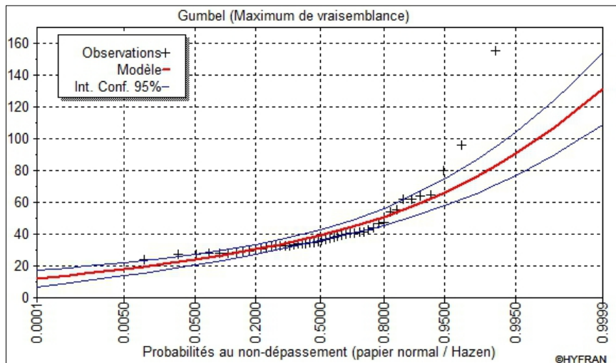
Figure 8: Ajustement de la loi de Gumbel sur le bassin versant de l'Ouémé à Bétérou
