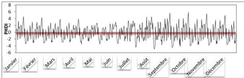
Figure 4 : Indices de sécheresse hydrologique de Palmer (PHDI)
